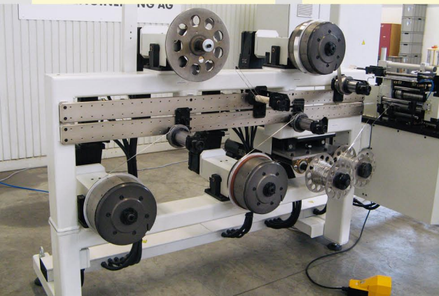
Общий вид блока намотки с индивидуально регулируемыми элементами
