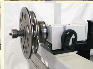
^ Намотка на барабаны, шпули, гильзы или кассеты с возможностью регулирования ^ силы натяжения намотки от 2 до 200 Н, возможна также фрикционная намотка диаметром от 76 до 600 мм
